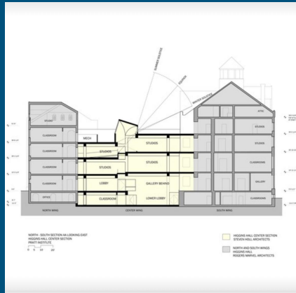
Longitude section
